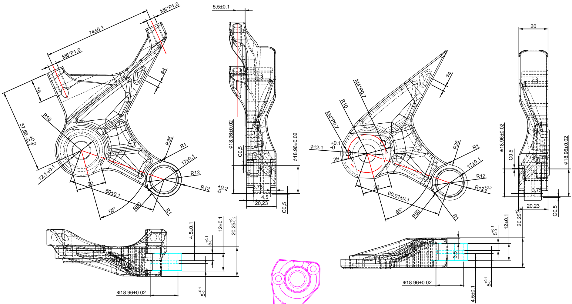
配9T-0101 吊耳
